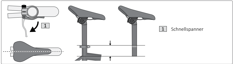
Abb. 18: Sattelhöhe einstellen (Klemmung mit Schnellspanner)
