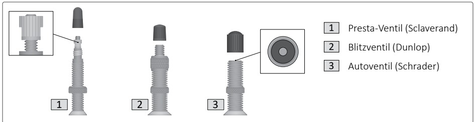
Abb. 17: Ventiltypen
