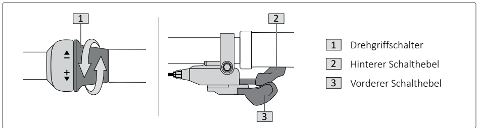
Abb. 14: Bedienelemente der Gangschaltung*
