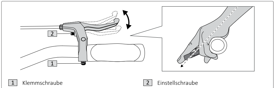
Abb. 12: Bremshebel einstellen
