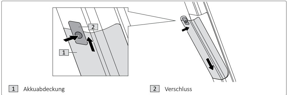
Abb. 8: Akkuabdeckung montieren
