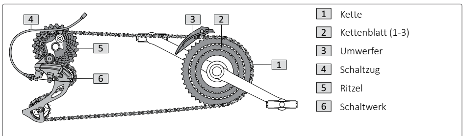
Abb. 15: Komponenten der Kettenschaltung
