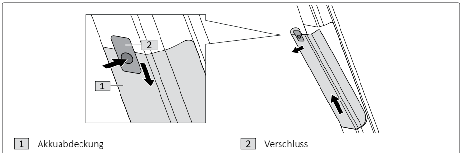
Abb. 6: Akkuabdeckung abnehmen
