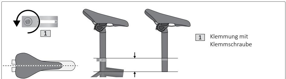
Abb. 19: Sattelhöhe einstellen (Klemmung mit Klemmschraube)
