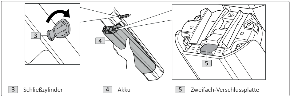
Abb. 7: Vollintegrierten Akku entnehmen/einsetzen
