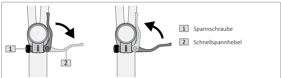
Abb. 24: Schnellspanner
