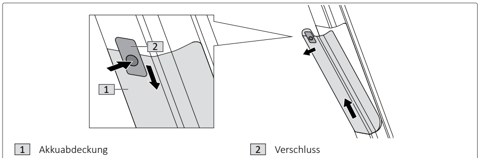
Abb. 6: Akkuabdeckung abnehmen
