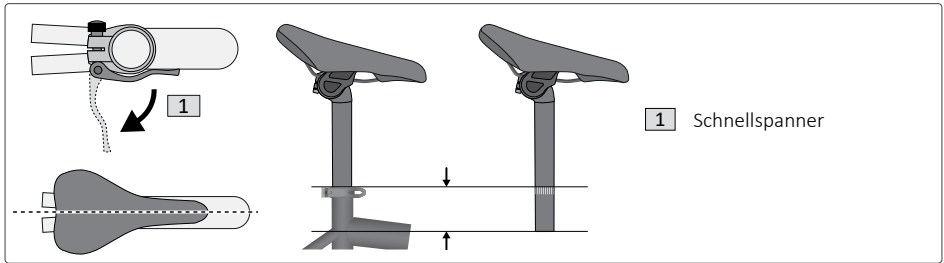
Abb. 14: Sattelhöhe einstellen (Klemmung mit Schnellspanner)
