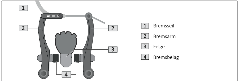
Abb. 7: Komponenten der Felgenbremse
