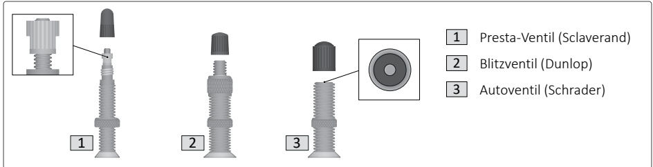
Abb. 13: Ventiltypen
