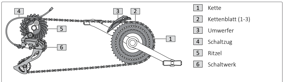
Abb. 11: Komponenten der Kettenschaltung
