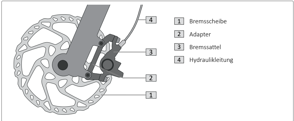
Abb. 6: Komponenten der Scheibenbremse
