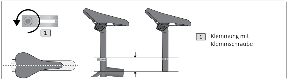
Abb. 15: Sattelhöhe einstellen (Klemmung mit Klemmschraube)
