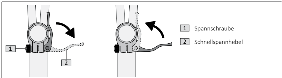
Abb. 20: Schnellspanner
