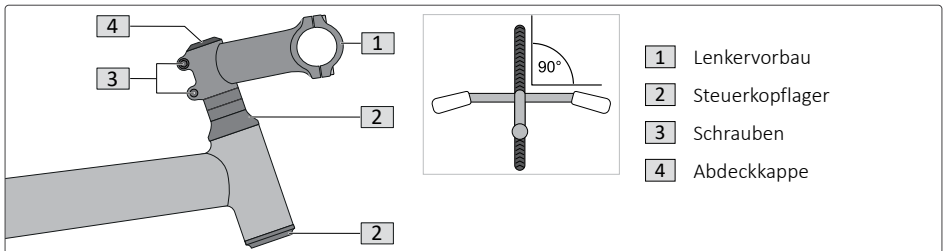
Abb. 17: Lenkervorbau einstellen (Klemmung mit Klemmschraube)
